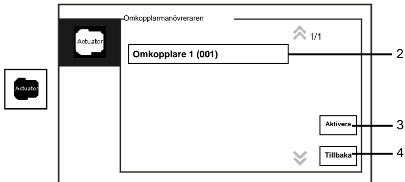
Fig. 12 Omkopplarmänövreraren
