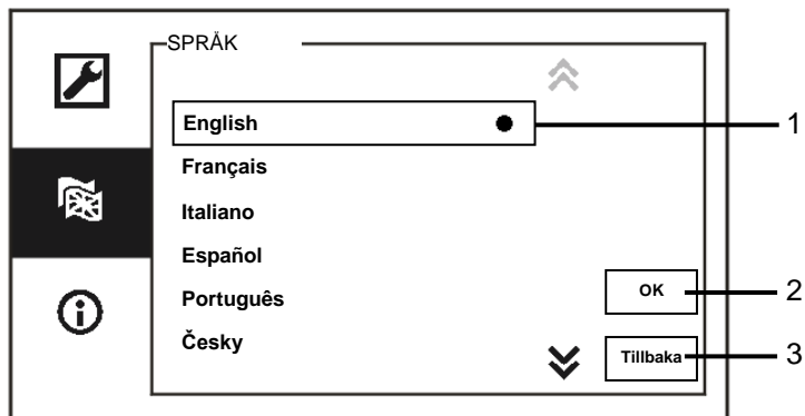
Fig. 22 Språkinställningar
