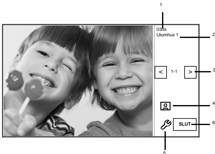
Fig. 3 Inkommande samtal
