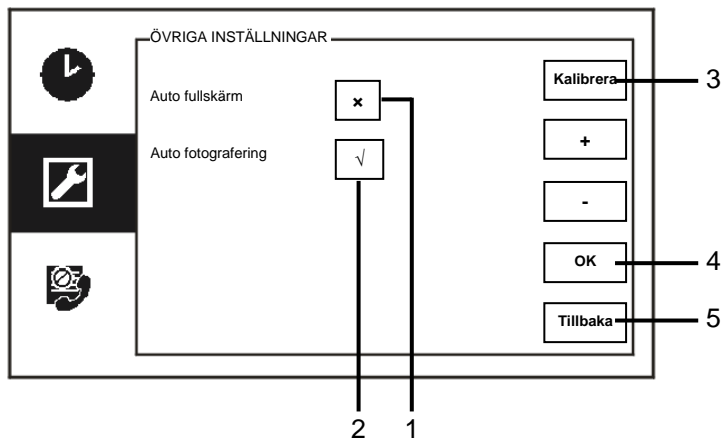
Fig. 21 Övriga inställningar
