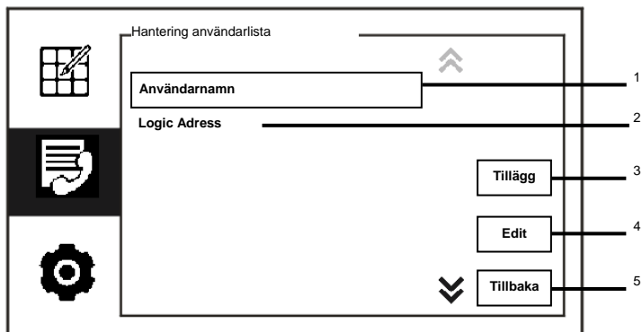
Fig. 28 Hantering användarlista
