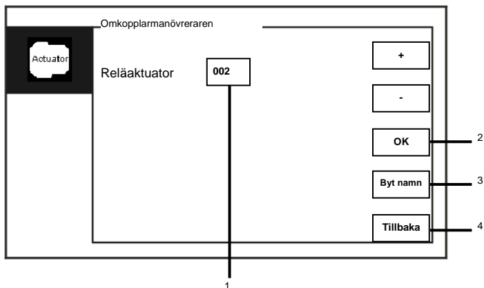
Fig. 26 Omkopplarmanöverarinställningar
