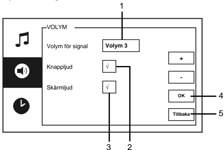
Fig. 19 Volyminställningar
