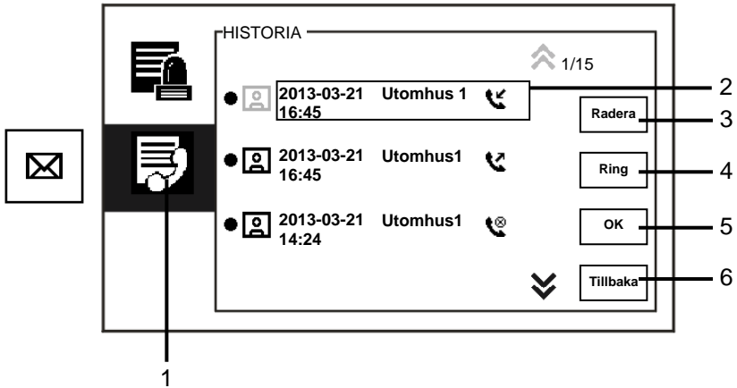
Fig. 15 Historia
