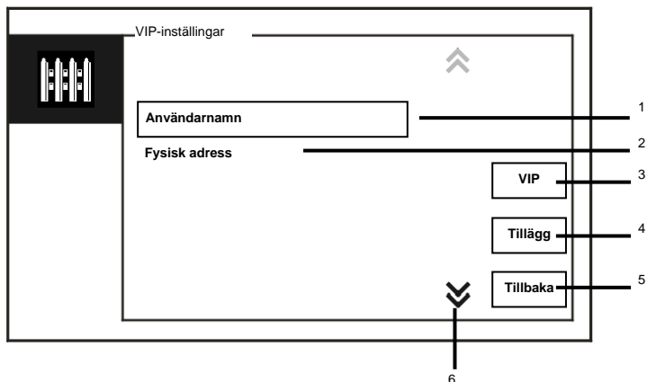
Fig. 6 VIP-inställningar
