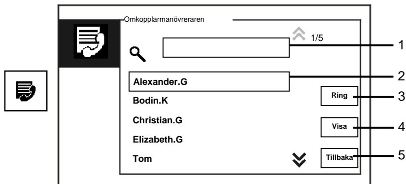
Fig. 13 Användarlista
