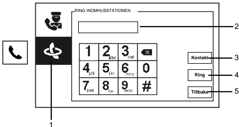
Fig. 9 Ring inomhusstation
