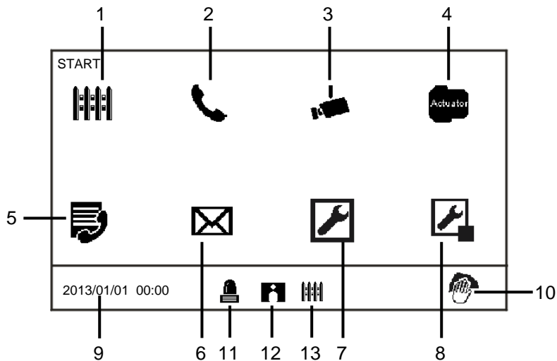
Fig. 2 Start
