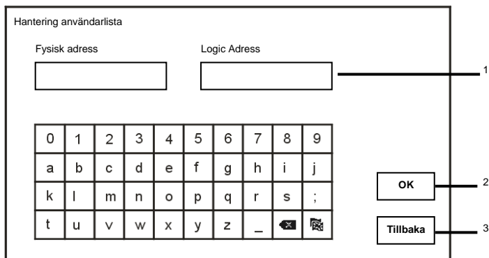
Fig. 31 Hantering användarlista
