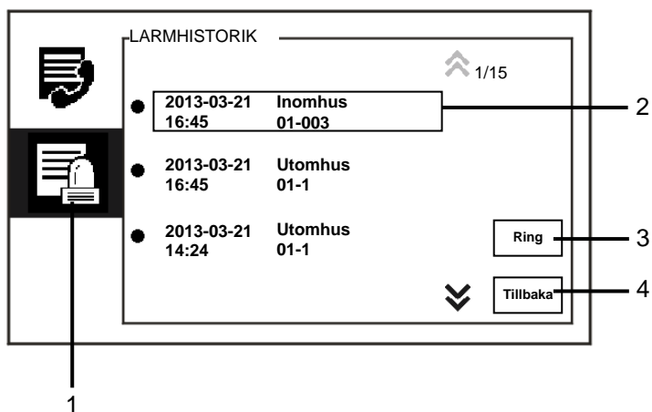
Fig. 17 Larmhistorik
