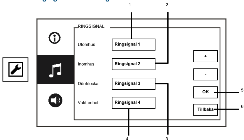
Fig. 18 Ringsignalsinställningar
