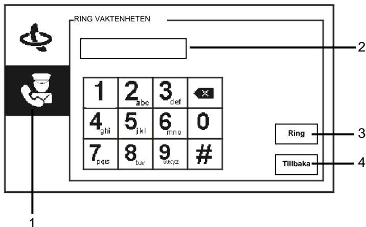
Fig. 10 RING VAKTENHETEN
