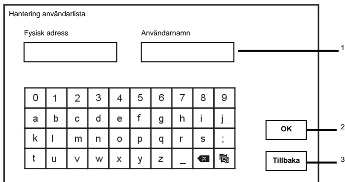
Fig. 29 Användarnamn
