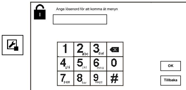
Fig. 24 Lösenord
