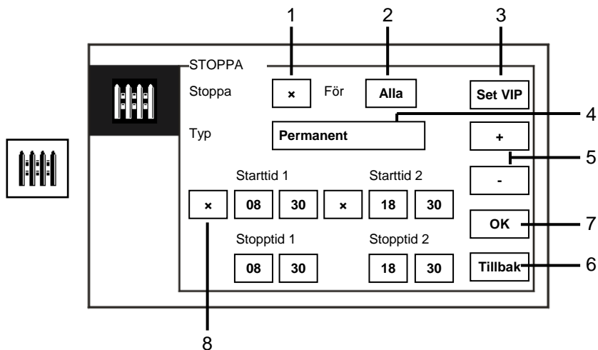
Fig. 5 Avlyssningsläge
