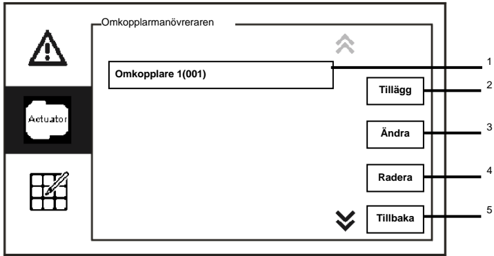
Fig. 25 Omkopplarmanövererinställningar
